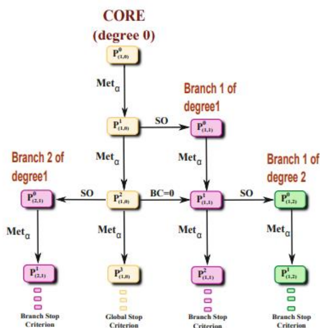
Gambar 4.4. 3 tingkat struktur pohon HGS-Sched
