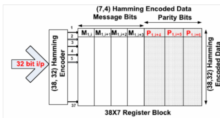
Gambar 7.14. Struktur skematis dari encoder H-PC yang diusulkan
