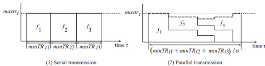
Gambar 3.14. Waktu transmisi
